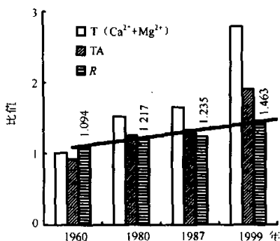
图2 太湖湖水总硬度对总碱度比值 随时间变化趋势曲线
