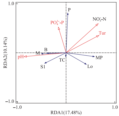
图5 丹江口水库丹库区浮游植物优势功能群与环境因子的RDA分析
