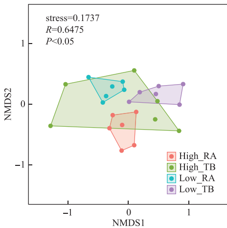
图4 丹江口水库丹库区浮游植物功能群组成不同时空下非度量多维排列分析
