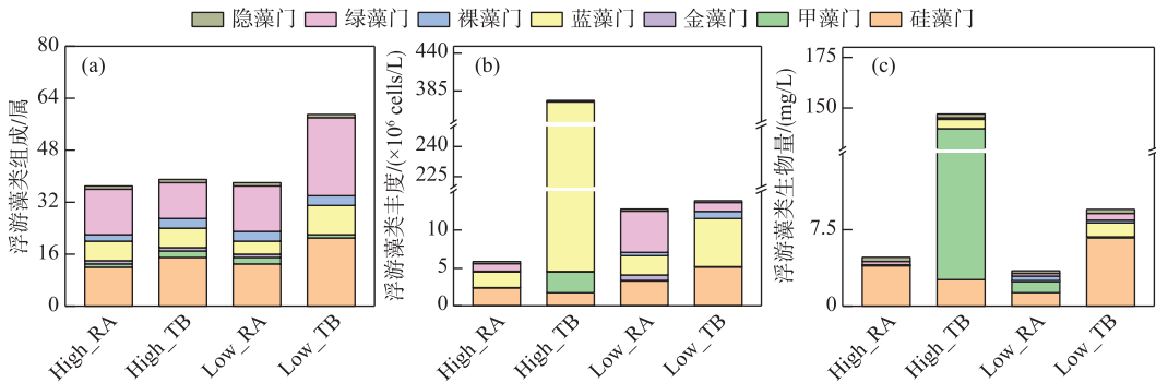
图 2 丹江口水库丹库区不同时空浮游植物组成(a)、丰度(b)和生物量(c)
