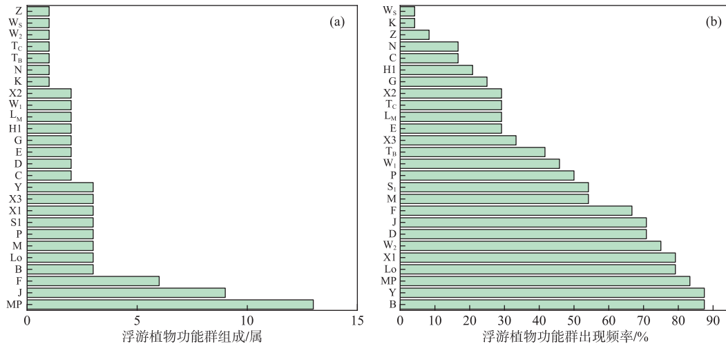
图3 丹江口水库丹库区浮游植物功能群组成(a)和出现频率(b)
